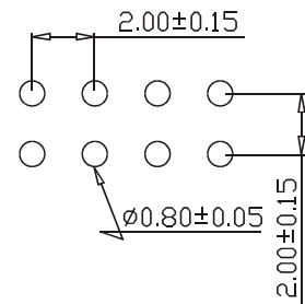
P.C.B LAYOUT
